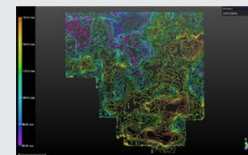
레이저스캔 기반 슬래브 평탄도 관리
